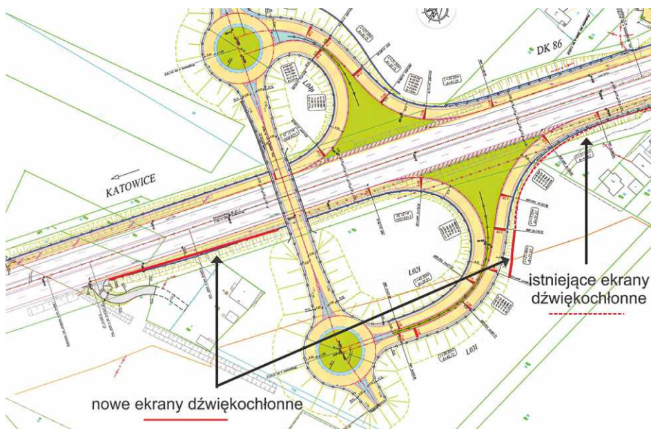
Mapka przedstawiająca rozmieszczenie ekranów dźwiękochłonnych
